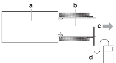
a Блок BS b Отводной воздуховод c Направление воздухоотока d Проволоочный термоанемометр
