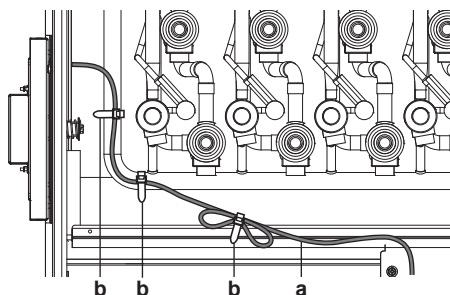
a Spjeldledning b Kabelbånd
