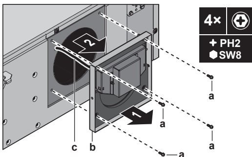
a Skruer b Spjeld c Spjeldledning
