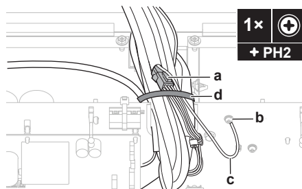
a Koblingsstykke b Skruer på jordledning c Jordledning til spjeld d Kabelbånd
