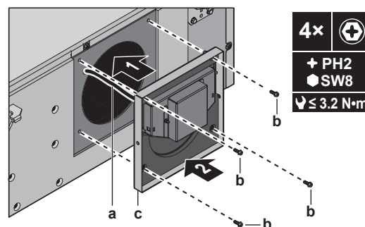
a Spjeldledning b Skruer c Spjeld
