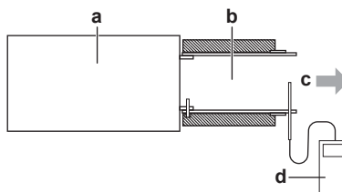
a BS unit b Luchtuitlaatkanaal c Luchtstroomrichting d Thermische anemometer
