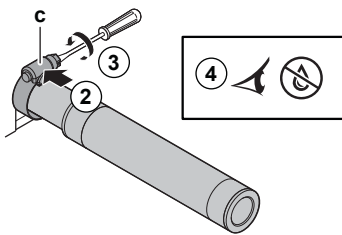
c Abrazadera de metal (accesorio)
