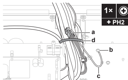
a Konektor b Šroub zemnicího vodiče c Zemnicí vodič klapky d Kabelová spona
