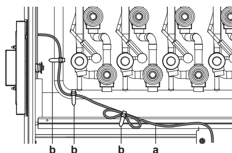
a Vodič klapky b Kabelová spona
