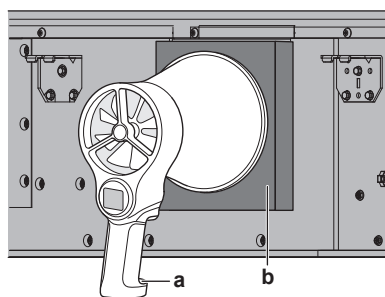
a Lopatkový anemometr b Sada pro připojení potrubního kanálu (EKBSDCK)
