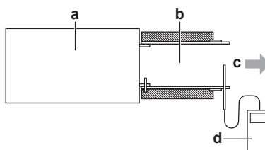
a Jednotka BS b Výstupní vzduchový kanál c Směr proudu vzduchu d Anemometr se žhavicím drátem
