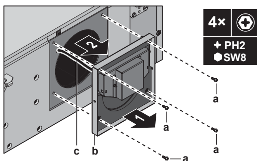
a Šroub b Klapka c Vodič klapky
