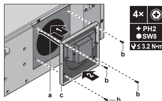
a Vodič klapky b Šroub c Klapka
