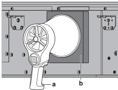
a Лопатков анемометър b Комплект за съединение на канал (EKBSDCK)
