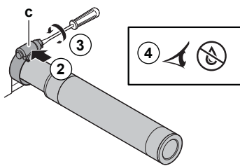
с Метална скоба (аксесоар)
