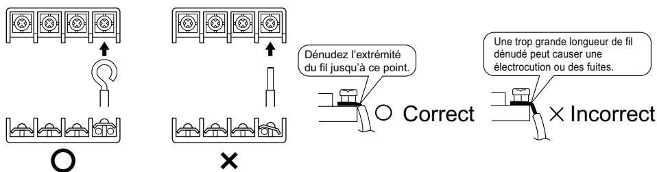
Fil dénudé sur le bornier de raccordement
