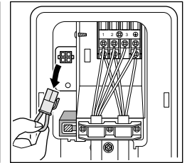
Bereitschafts-Stromsparfunktion EIN.
