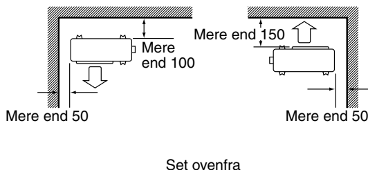
Væg på to sider
