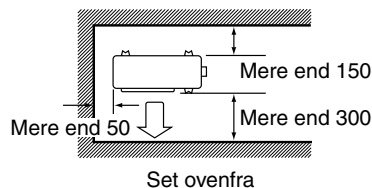
Væg på tre sider
