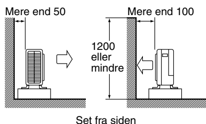
Væg på én side
