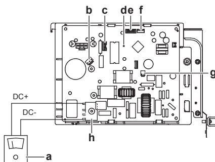
a Multimetricu (intervalul de tensiuni de curent continuu)
