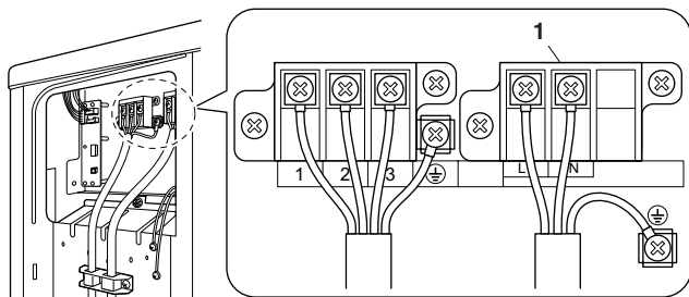
1 Svorkovnice napájení
