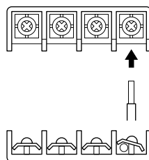
○ Kabels strippen bij het aansluitingsblok X
