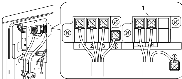
1 Tehonsyötön riviliitin
