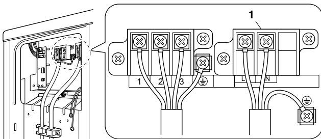
1 Kopplingsplint för spänningskälla
