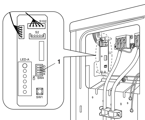
1 Aktivera brytare B
