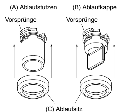
(C) Ablaufsitz
