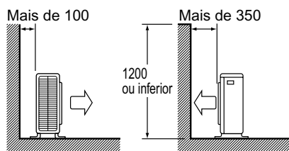
Vista lateral
