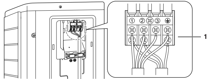
1 Strømforsynings klemrække
