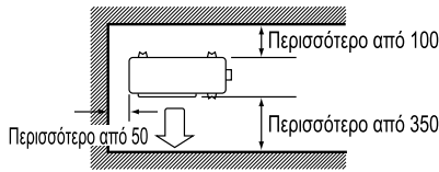
Πάνω όψη
