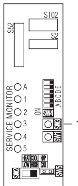
1 Johdotusvirhetarkastuskytkin SW3
