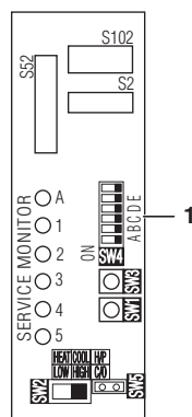
1 Kontakt Indstilling af prioriteret rum (SW4)
