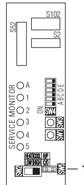
1 Kontakt til indstilling af Støjsvag drift nat SW5
