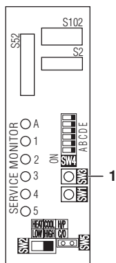
1 Stikalo za preverjanje napak v ožičenju (SW3)
