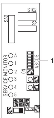
1 Sklopka za podešavanje za prioritetnu prostoriju SW4
