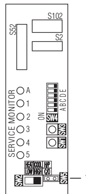
1 Sklopka za Night Quiet (tihi noćni) način rada SW5
