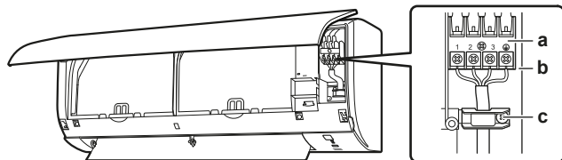
a Клеммная колодка b Распределительная коробка c Кабельная стяжка
