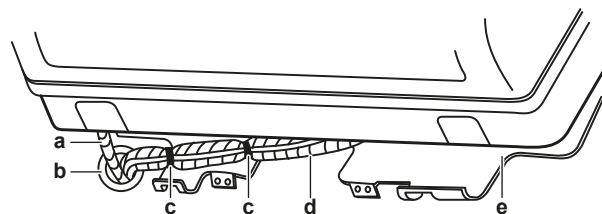
a Сливной шланг b Заделайте это отверстие мастикой или замазкой c Виниловая клейкая лента d Изоляционная лента e Монтажная пластина (входит в комплект принадлежностей)
