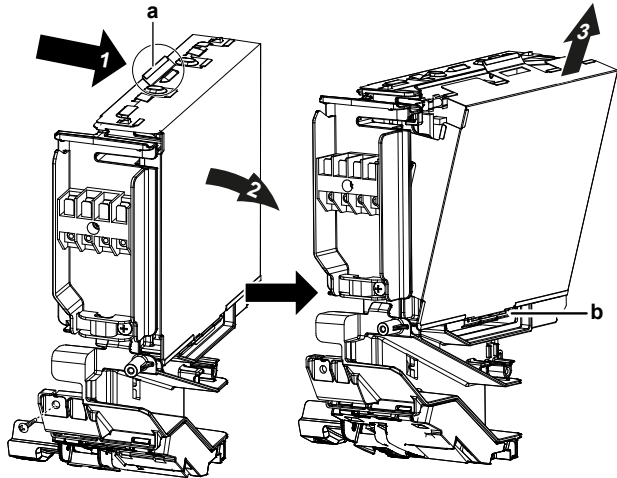
a Kannen päällä oleva ulkoneva osa b Kieleke
