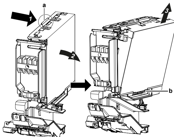
a Προεξέχον τμήμα στο πάνω μέρος του καλύμματος b Γλωττίδα
