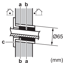
a Tubo incassato nella parete b Mastice c Copertura del foro nella parete
