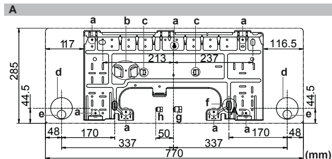
A Piastra di montaggio per le classi 25~35 a Punti di fissaggio consigliati per la piastra di montaggio b Tasca per il coperchio della porta del tubo c Linguette per posizionare la livella d Foro passante nella parete Ø65 mm e Posizione del tubo flessibile di scarico f Posizione per il metro a nastro sul simbolo ">" g Estremità del tubo del gas h Estremità del tubo del liquido
