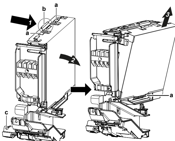
a Scheda b Parte sporgente in cima al coperchio c Vite
