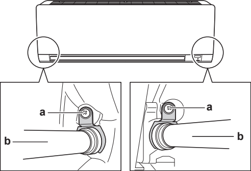
a Tornillo de fijación del aislamiento b Manguera de drenaje
