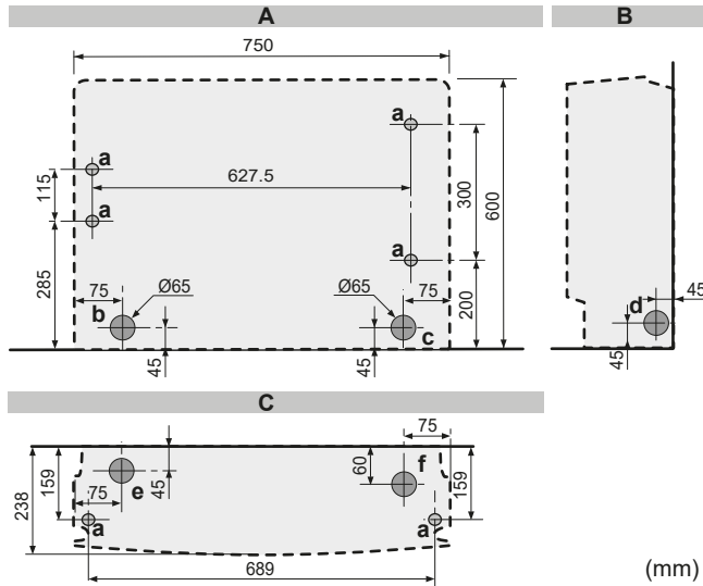
5-1 Цртеж за инсталирање на внатрешна единица: Подно-парапетна инсталација
