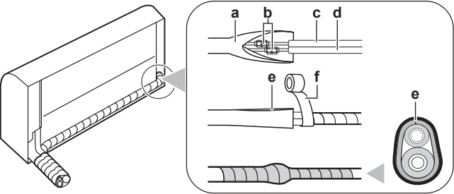
a Оболонка теплоізоляційної трубки (на боці внутрішнього блоку)
