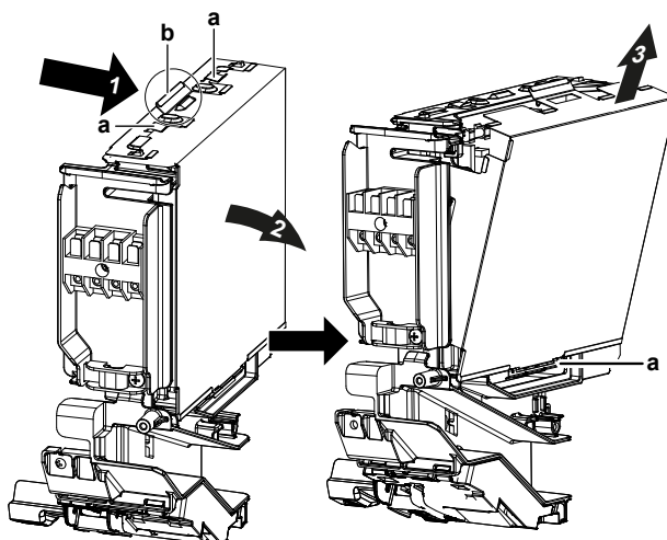
a Язычок b Верхняя выступающая часть крышки распределительной коробки
