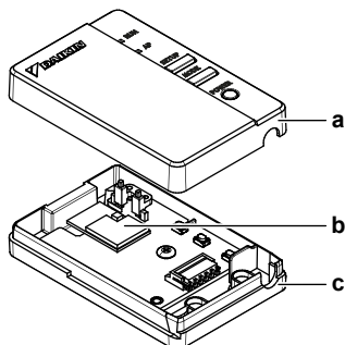
а Горно кукиште б Печатена плоча на безжичниот ЛАН-адаптер с Долно кукиште
