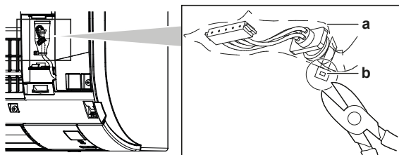
а Заштитна обвивка б Стега
