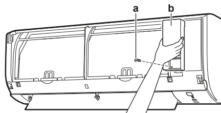
a Винт сервисной крышки b Сервисная крышка
