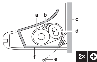
a Сливной шланг b Соединительный кабель c Монтажная пластина (входит в комплект принадлежностей) d Трубопровод хладагента e Крепежный винт M4x12L внутреннего блока (входит в комплект принадлежностей) f Нижняя рама
