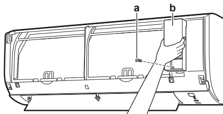
a Skruv för serviceluckan b Servicelucka
