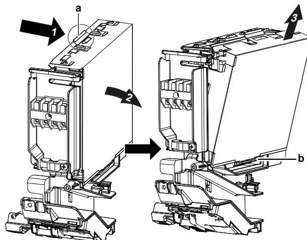
а Верхняя выступающая часть крышки распределительной коробки б Язычок
