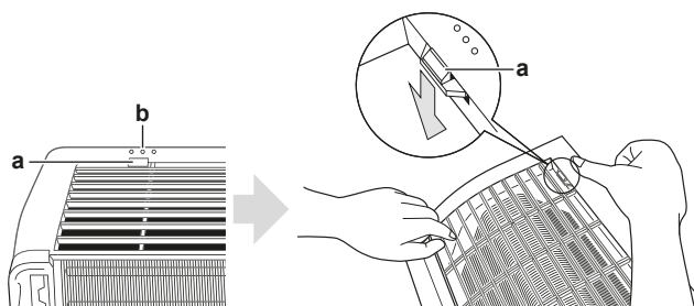
а Верхний крючок б Значок с 3 окружностями
