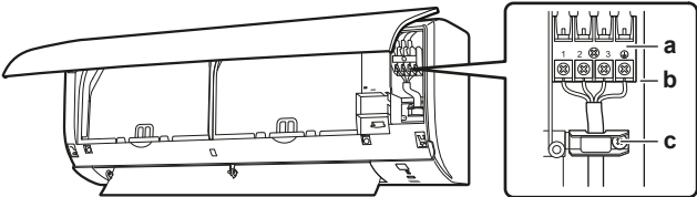
a Listwa zaciskowa b Skrzynka podzespołów elektrycznych c Zacisk kablowy
