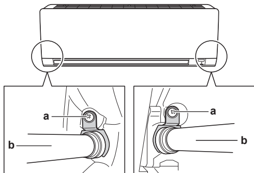
a Șurub de fixare a izolației b Furtun de evacuare
