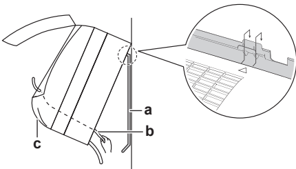
a Placa de montaje (accesorio) b Cable de interconexión c Guía de cables
