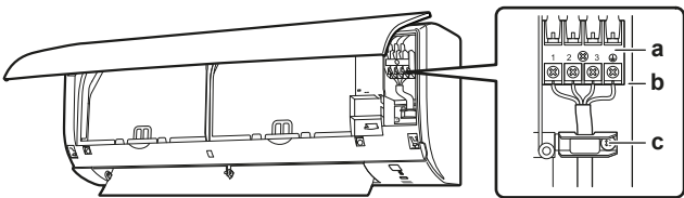
a Bloque de terminales b Bloque de componentes eléctricos c Abrazadera para cable
