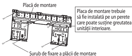
Punctele de fixare recomandate și dimensiunile plăcii de montare
