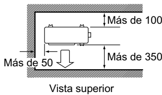
Vista superior
