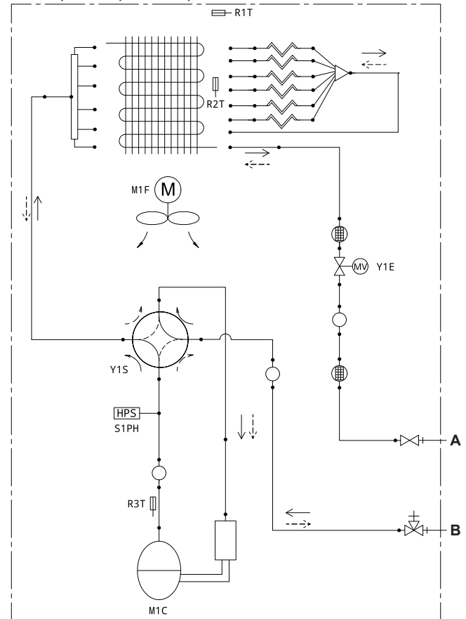
Легенда на дијаграм за поставување цевки
