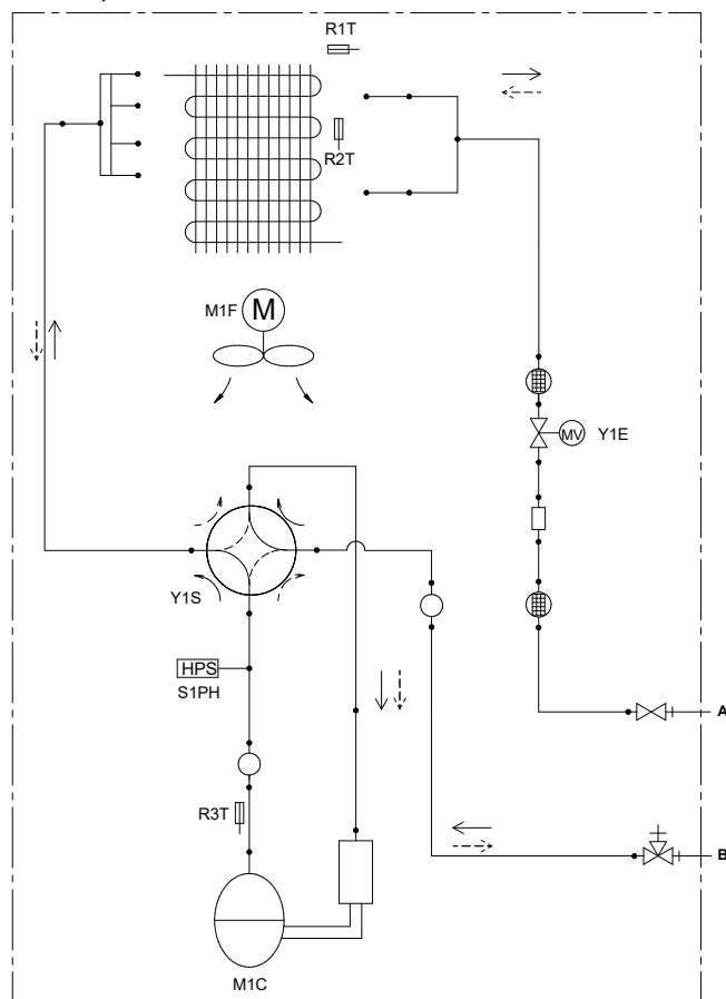
Легенда на дијаграм за поставување цевки
