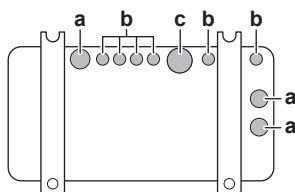
a Dräneringshål. Installera ett dräneringslock (stort). b Dräneringshål. Installera ett dräneringslock (litet). c Hål för dräneringsfästet
