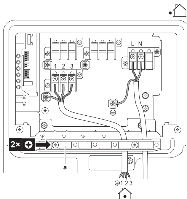
a Držač žice
