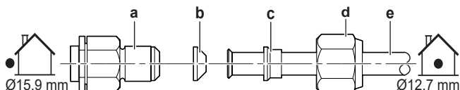
a Ștuț de racordare al unității exterioare
