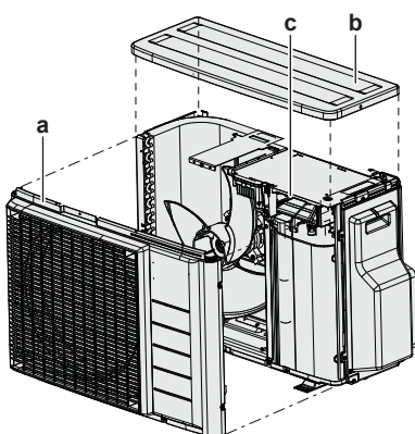
a Frontplåt b Överdel c S99-kontakt
