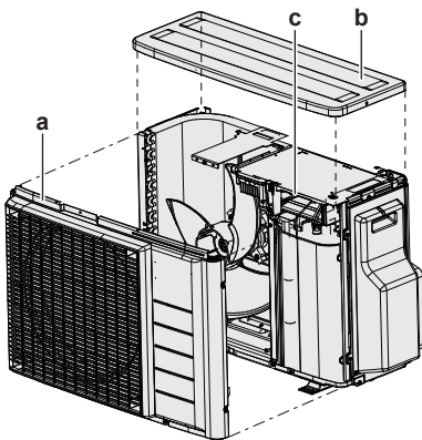
a Čelna plošča b Zgornja plošča c Konektor S99
