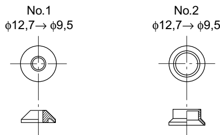
Empaquetadura (1)
