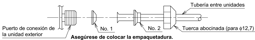
Empaquetadura (1)
