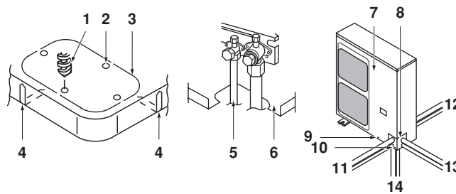
Rysunek - Przewody zewnętrzne prowadzone w czterech kierunkach
