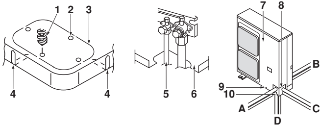
Obrázek - Provozní potrubí ve čtyřech směrech
